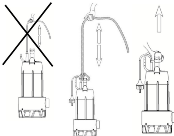
Abb. 5-2: Positionierung
