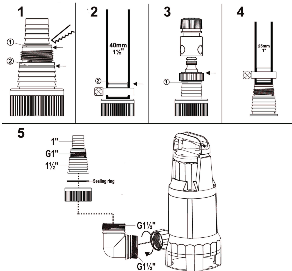
Abb. 5-3: Schlauchanschluss
