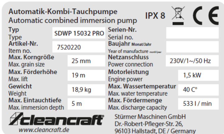
Abb. 2-1: Typenschild SDWP 15032 PRO
