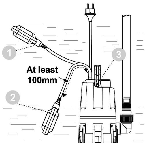
Abb. 5-1: Funktionsprinzip des Schwimmerschalters
