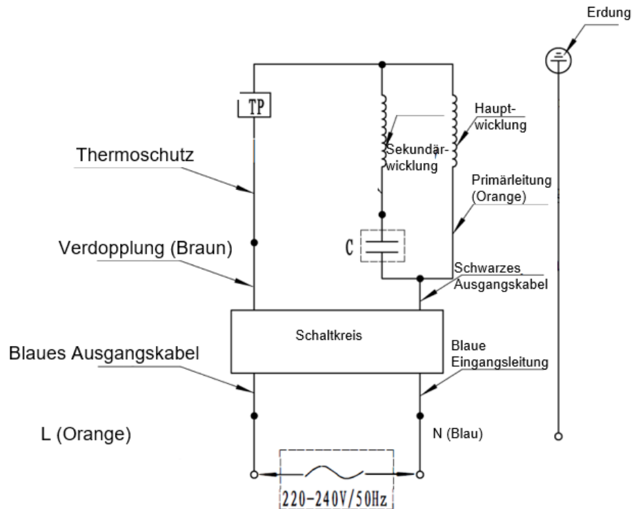
Abb. 10-1: Schaltplan SDWP 7514 A
