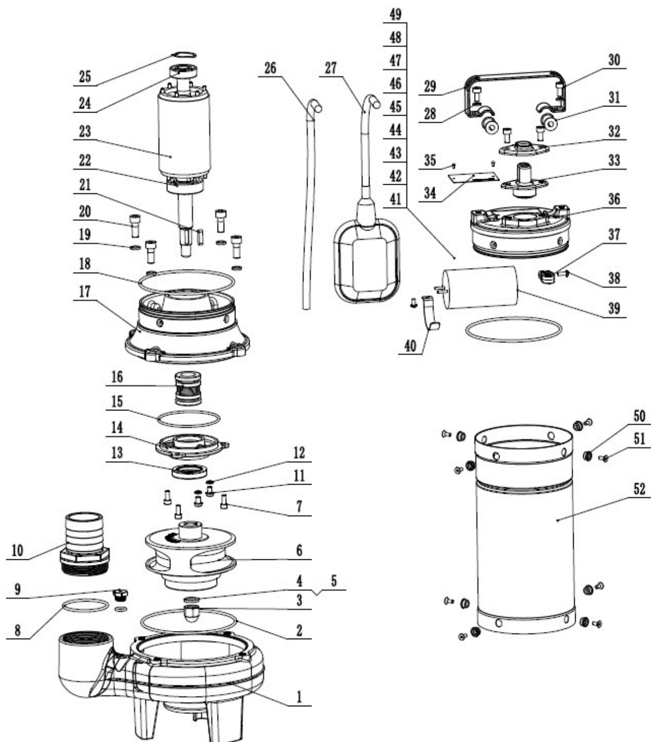
Abb.9-2: Ersatzteilzeichnung SDWP 15032 PRO
