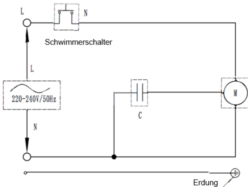
Abb. 10-2: Schaltplan SDWP 15032 PRO
