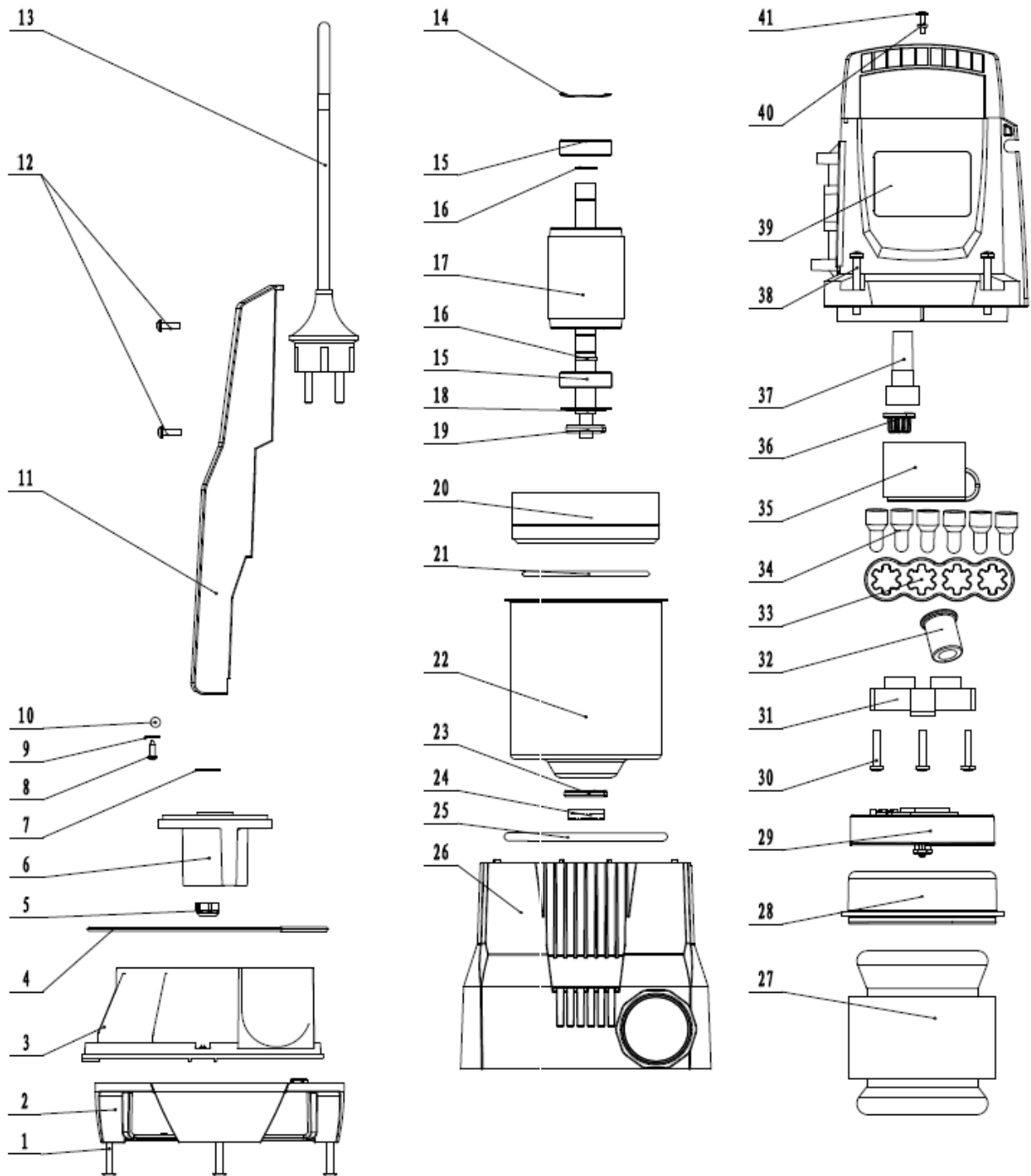
Abb. 9-1: Ersatzteilzeichnung SDWP 7514 A
