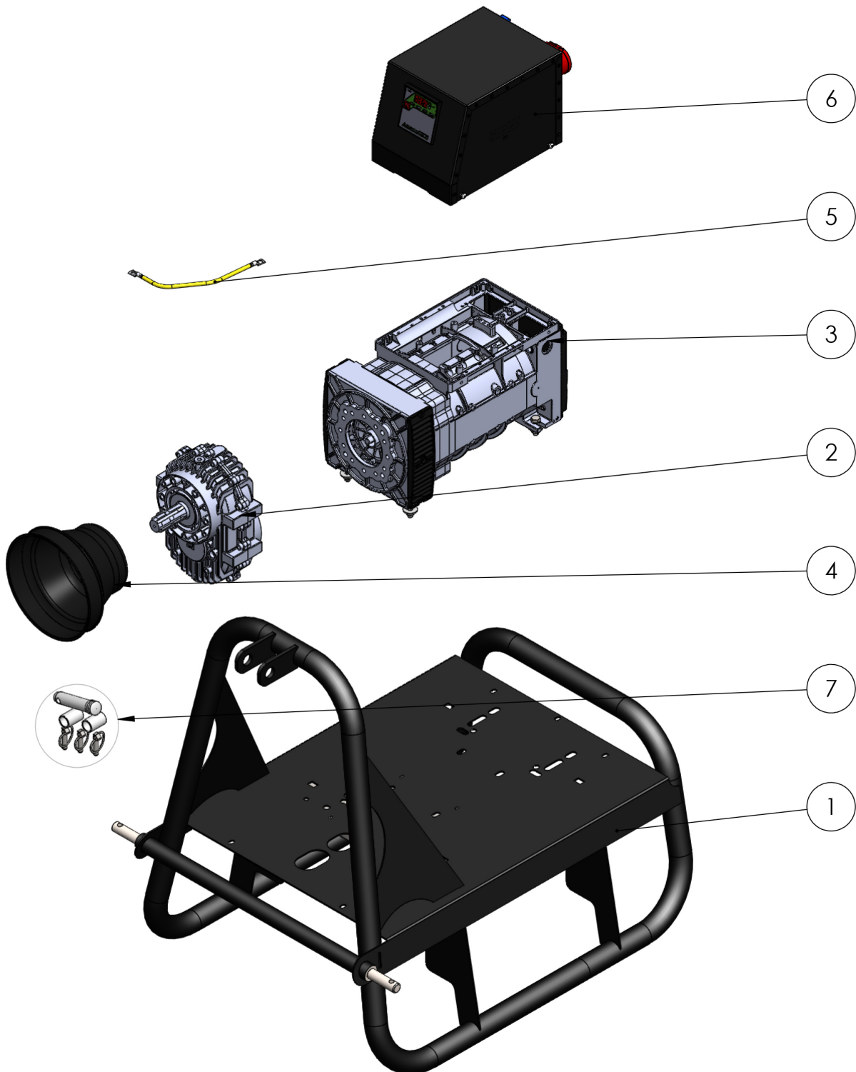
Abb. 8-1: Ersatzteilzeichnung 1
