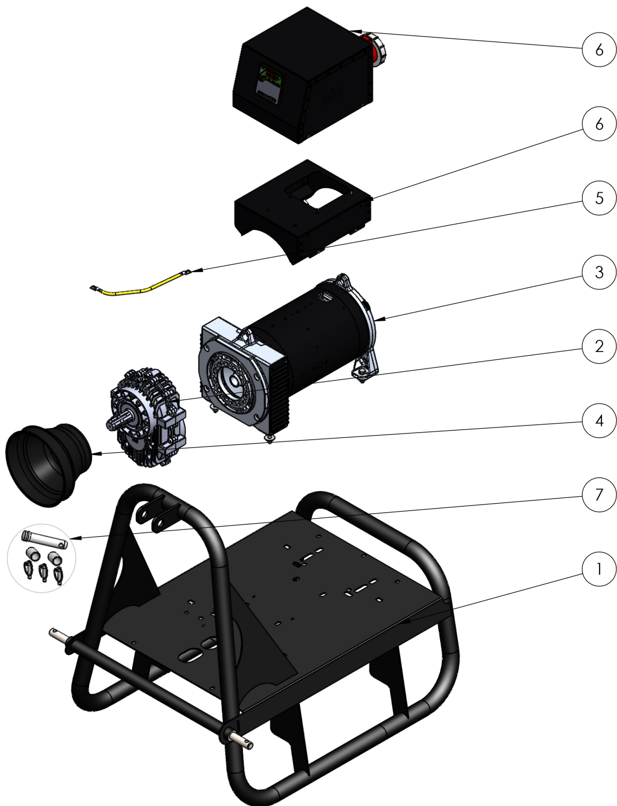
Abb.8-2: Ersatzteilzeichnung 2
