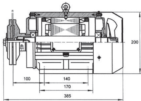
KRN mit Sägeblattflansch
