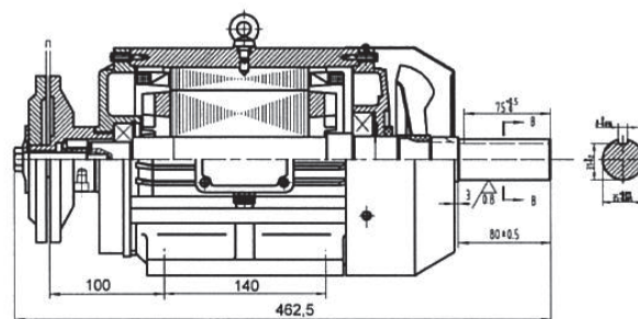
KRN mit Sägeblattflansch und zweitem Wellenende
