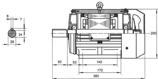
KRG mit Normwelle
