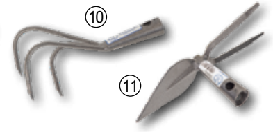
10 Grubber mit 3 Zinken aus hochwertigem Stahl und robuster Dülle. Arbeitsbreite von 14cm. Bestens geeignet für die Bodenbearbeitung. Best. Nr. K 114409 EUR 7,99
