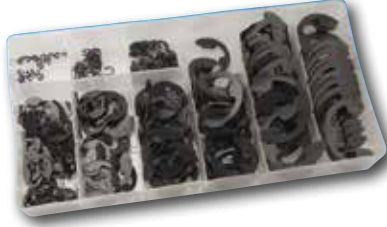
4 Sicherungsscheiben Sortiment, 300-tlg. Für Wellen mit Nut von 1,5 - 22 mm Nenn-Ø, 9 Größen, Federstahl, phosphatiert. Best. Nr. K 54314 EUR 17,95
